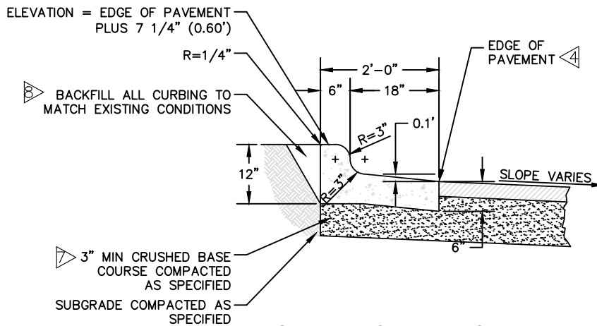
STANDARD "SPILL" TYPE CURB
